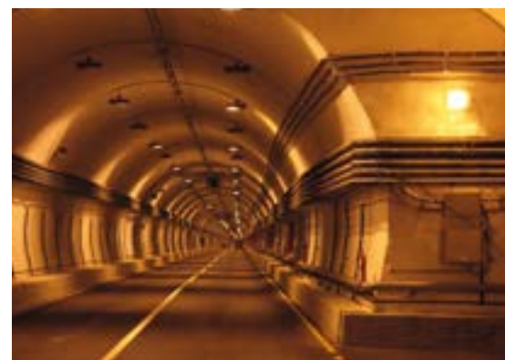
2010 г, р. Дагестан, Гимринский АДТ. Защита свода тоннеля антикарбонизационным покрытием MasterProtect 320 RAL 9010
